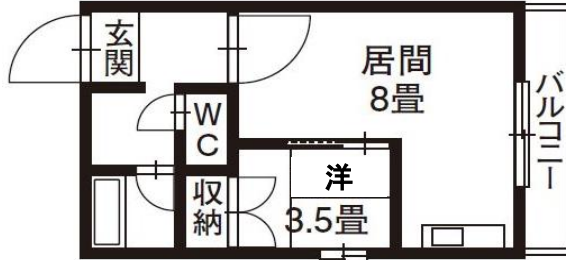
【間取り図】
